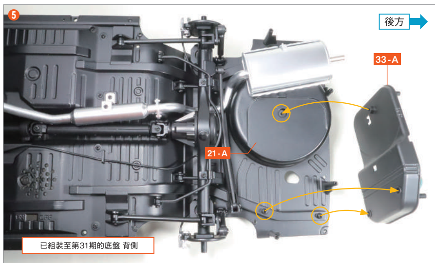
備妥已經組裝至第31期的底盤，將後地板面板 21-A 和油箱上部 33-A 的突起部分和凹槽對準然後嵌入。
