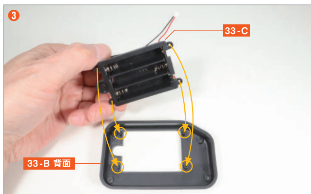
將 33-C 的4個凹槽與油箱下部 33-B 背面的4個螺絲孔突起部分對齊，然後將其嵌入。
