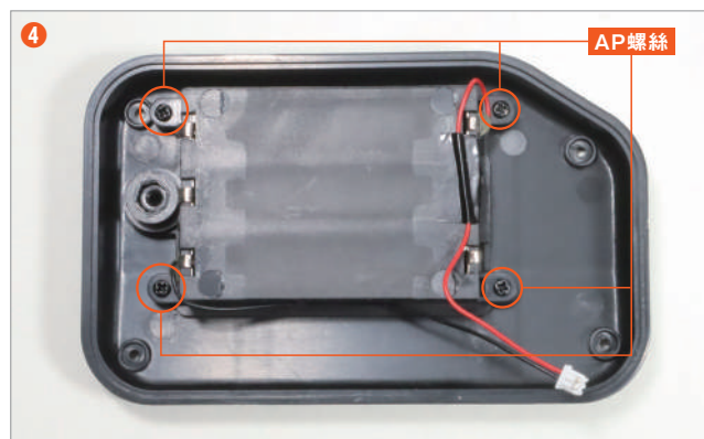
使用 AP 螺絲 固定4個位置。
